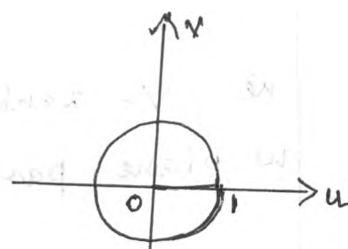
w -plane
