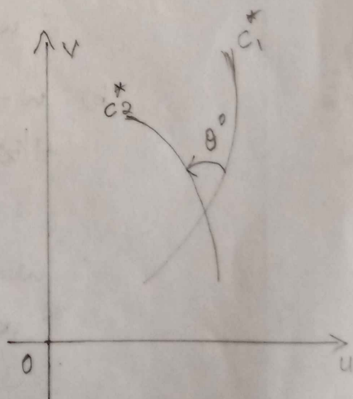
w -plane
