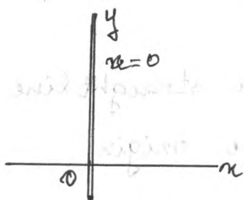
z -plane
